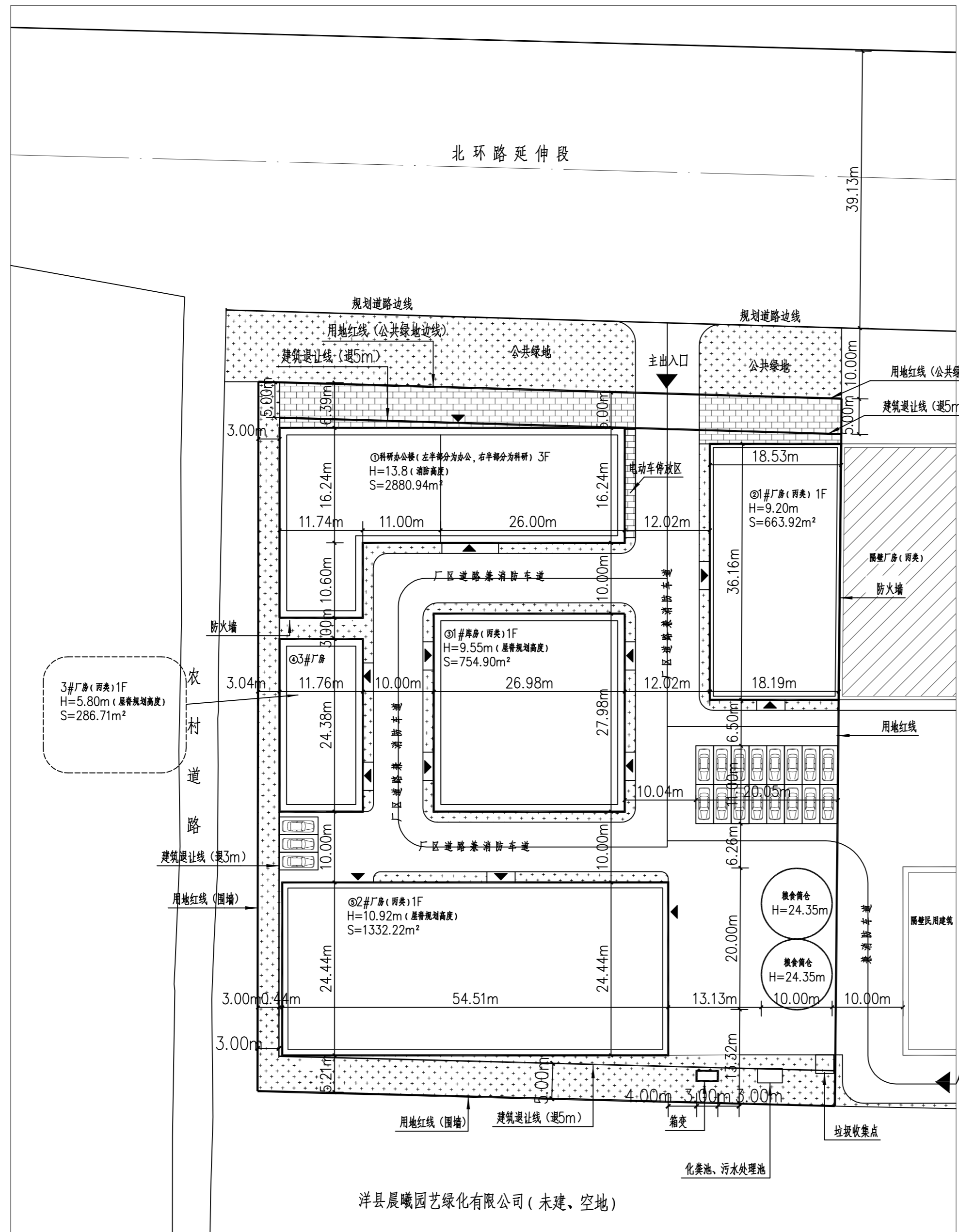
总平面图 1:500
